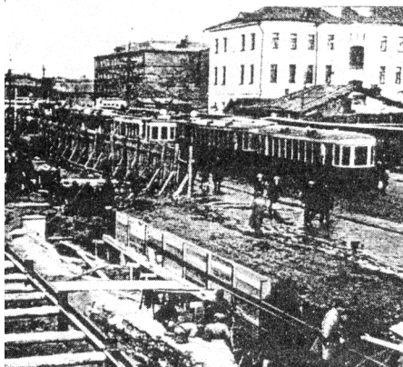
Строительство первой линии метрополитена
