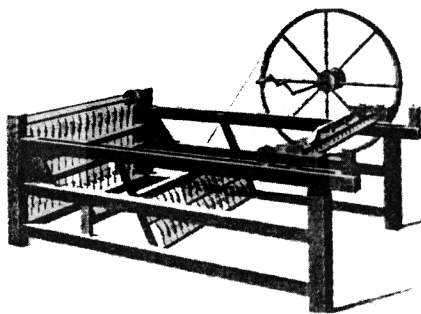
Прядильная машина «Дженни»
