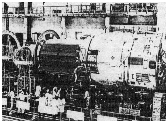
Орбитальная научная станция «Мир» во время наземной подготовки
